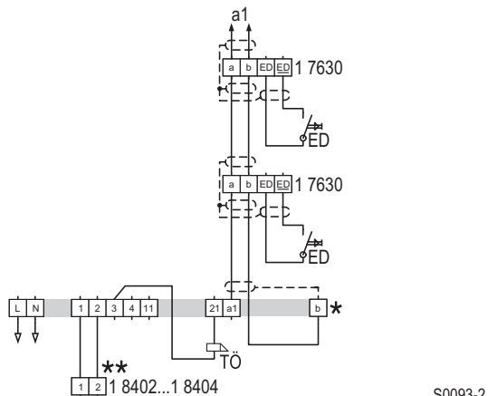
Schaltplan: Türsprechanlage für das Mehrfamilienhaus.
