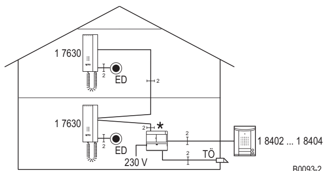
Blockschaltbild: Türsprechanlage für das Mehrfamilienhaus.
