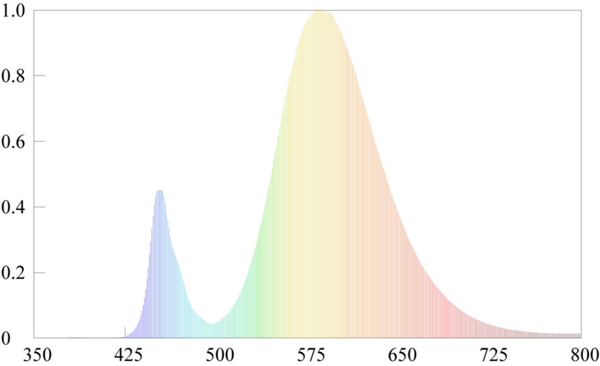
光谱分布 Spectral Distribution
