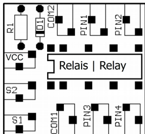
Fig. 1: Plan d'implantation
