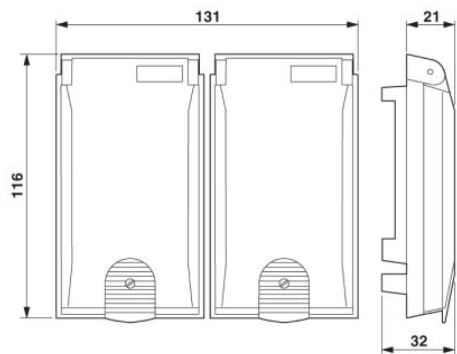
Cadre d'encastrement
